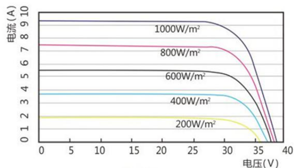
I-V 曲线
