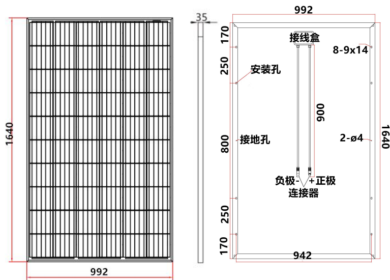
组件尺寸
